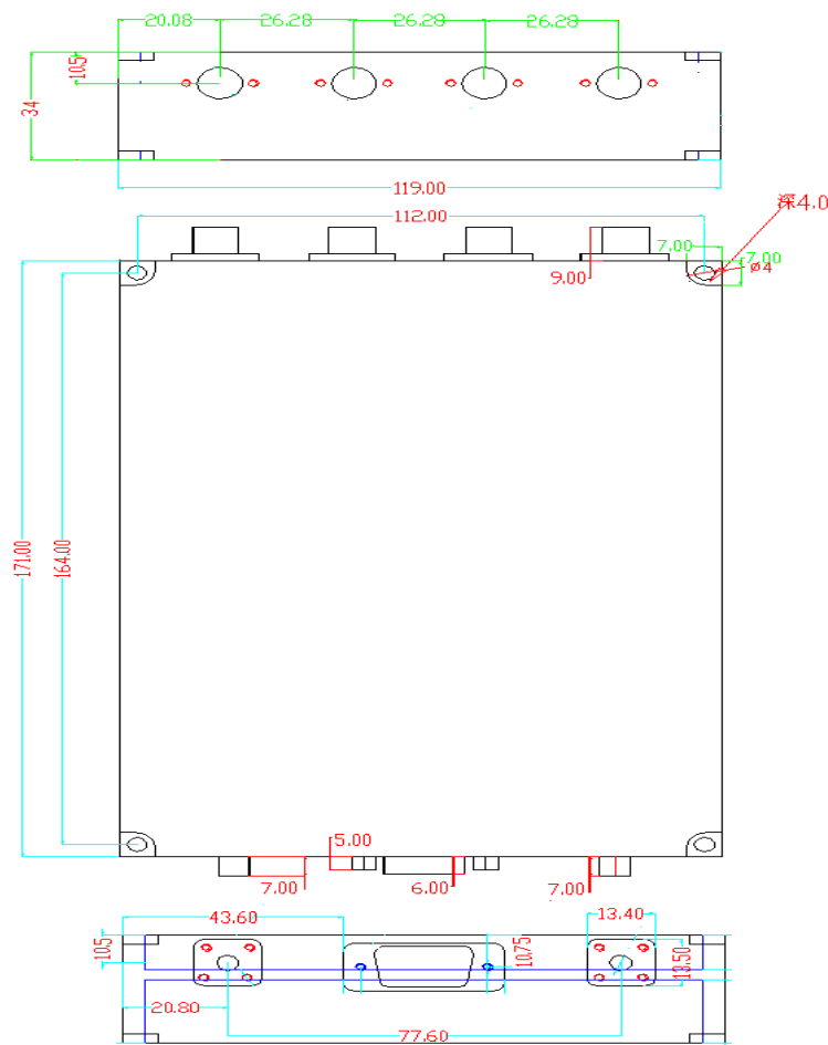
BST8815-XX
